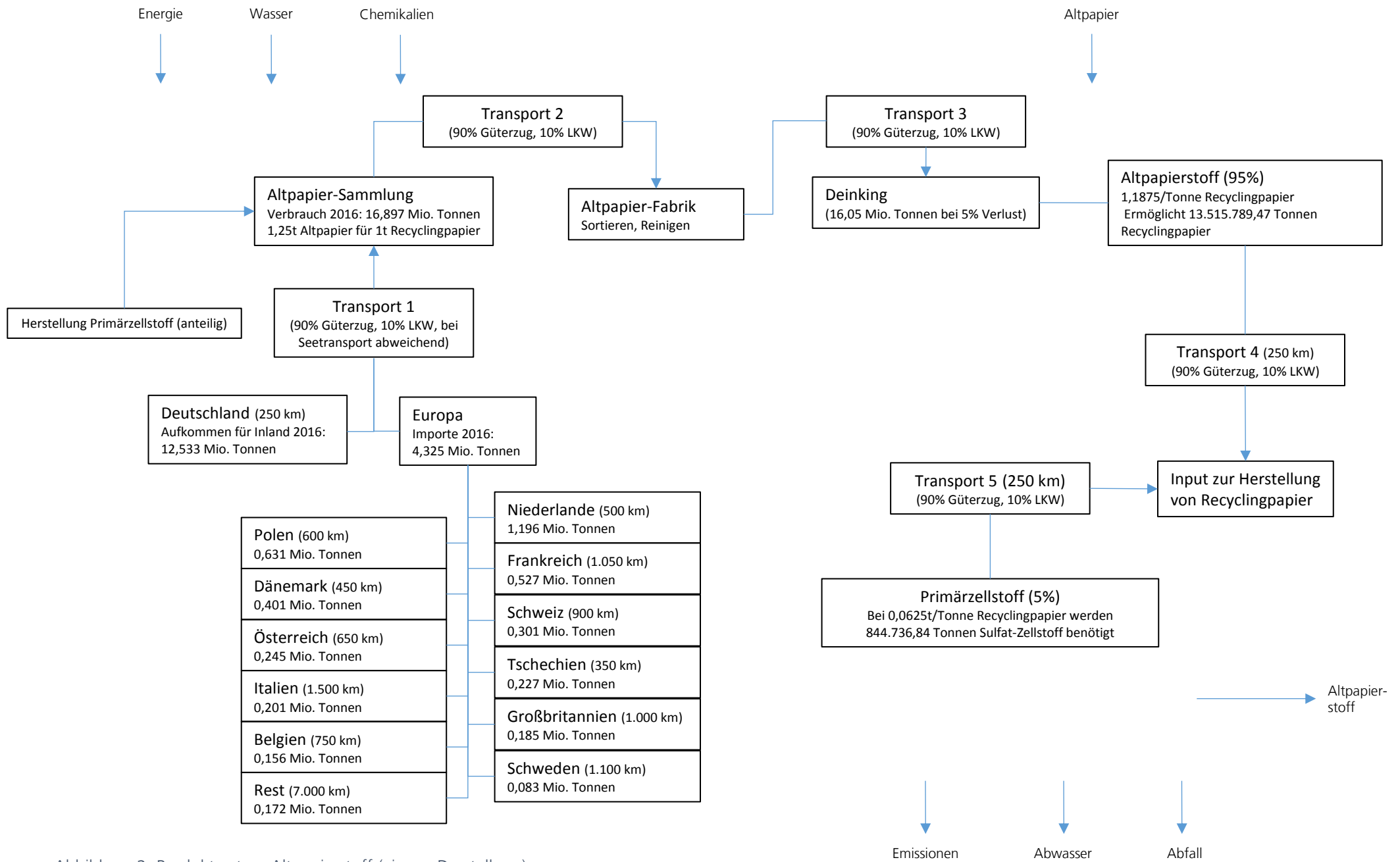
Abbildung 2: Produktsystem Altpapierstoff (eigene Darstellung).
