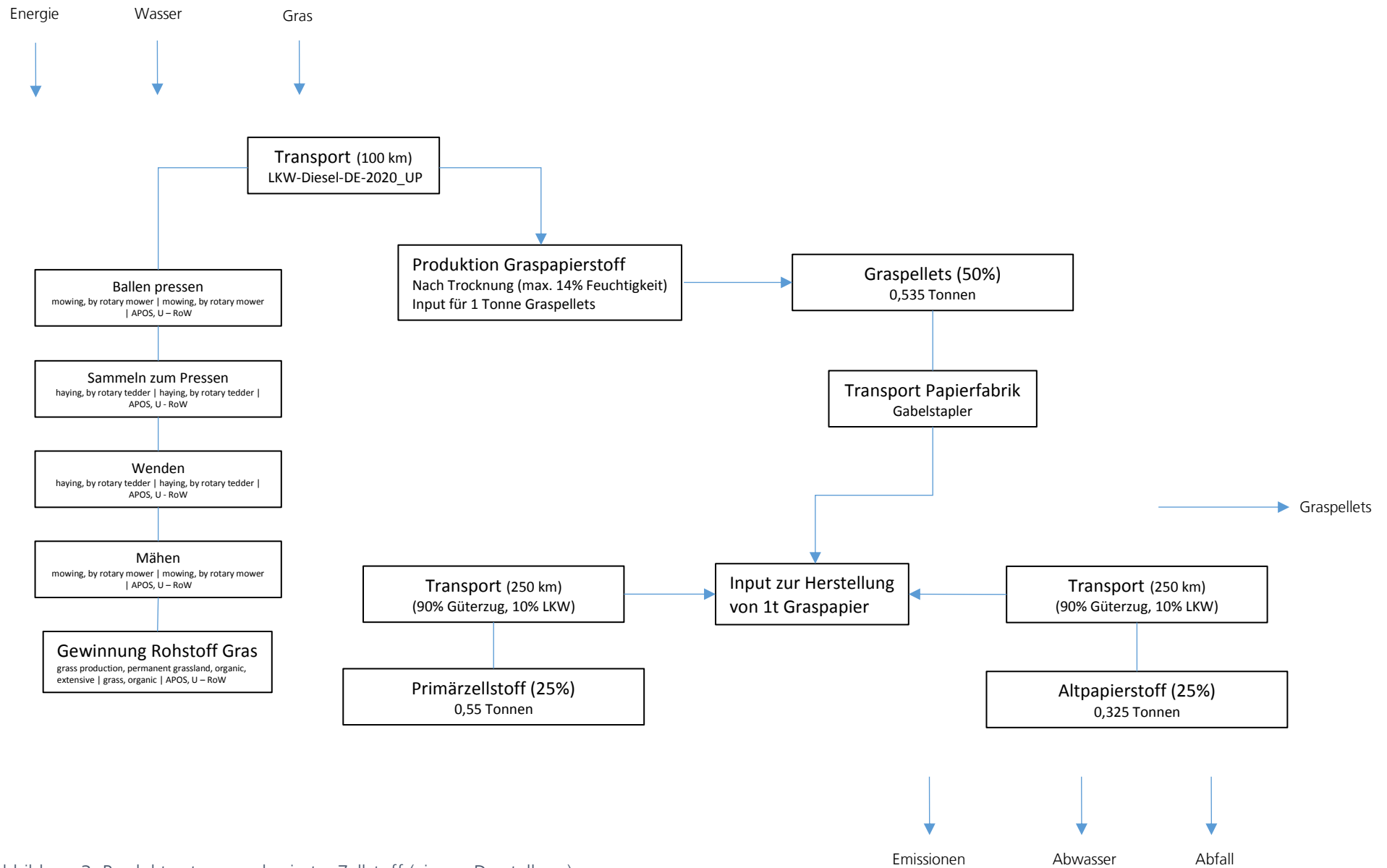
Abbildung 3: Produktsystem grasbasierter Zellstoff (eigene Darstellung).
